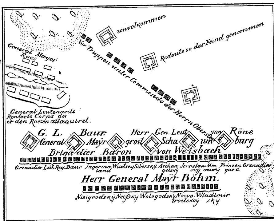
Боевой порядокъ русской конницы въ сраженіи подъ Полтавою 27-го Іюня 1709 года. Ярославскій драг. полкъ обозначенъ черною краскою.
